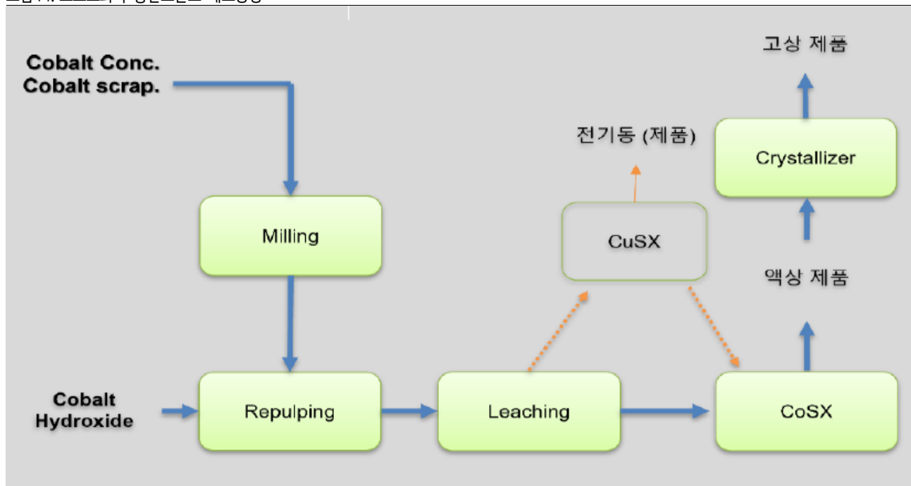
그림44. 코스모화학 황산코발트 제조공정
