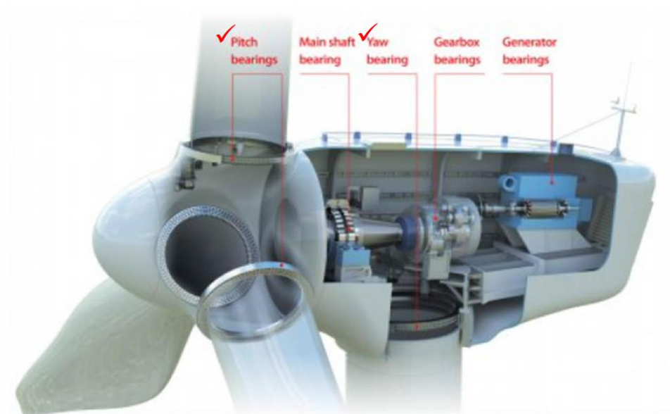
그림31. Pitch(Blade) &amp; Yaw Bearing in WTG
