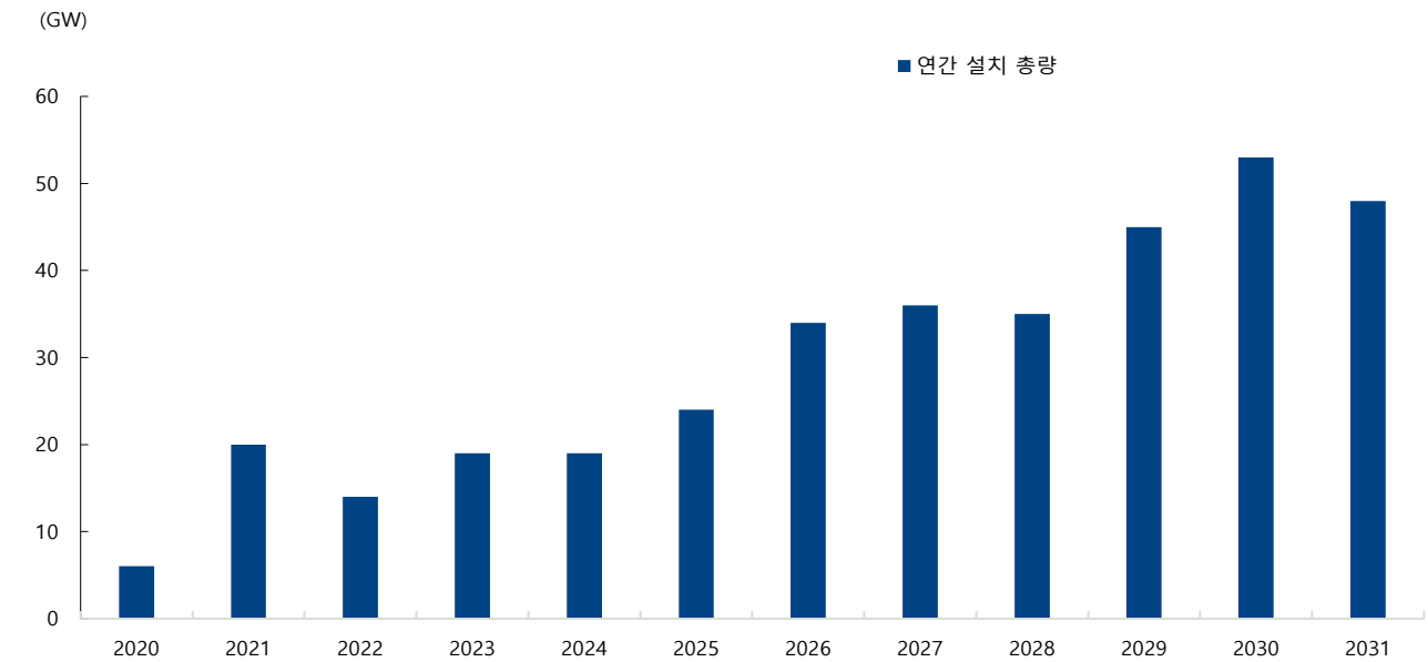
그림60. 글로벌 해상풍력 설치량 현황 및 전망
