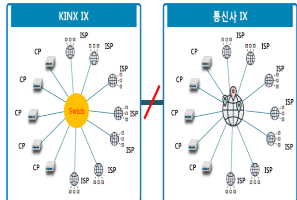
그림40. 중립적 인터넷회선연동 (IX) 서비스
