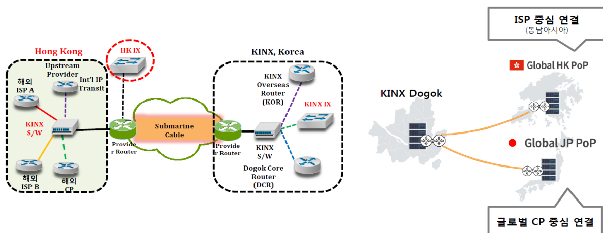
그림41. 인터넷회선연동 (IX) 서비스 확장
