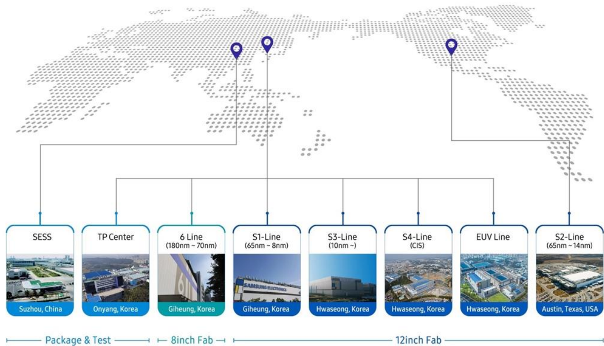
그림 6. 삼성전자 System LSI Foundry 현황
