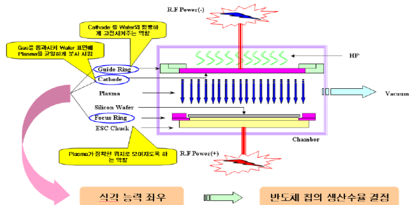
그림5. 에칭 공정도
