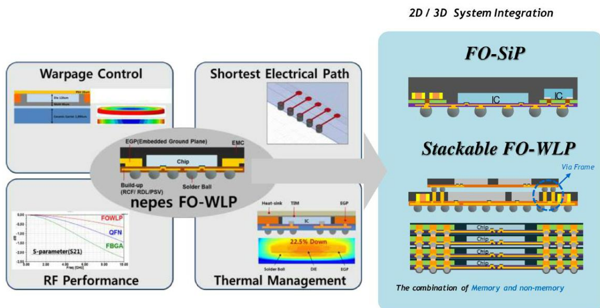
그림51. FOWLP(Fan-out WLP)
