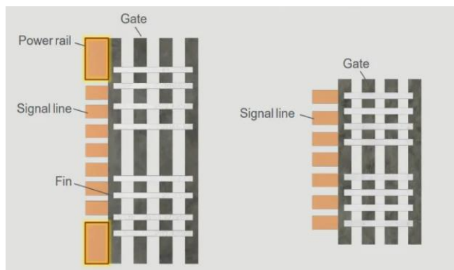
[그림 04] BSPDN 기술 도입으로 20~30% 수준의 공간 확보 가능 (2)
