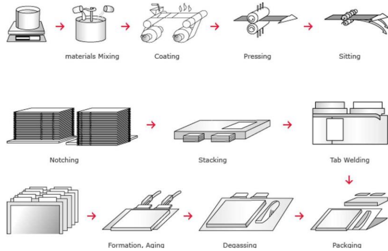
그림1 파우치타입 배터리 제조과정
