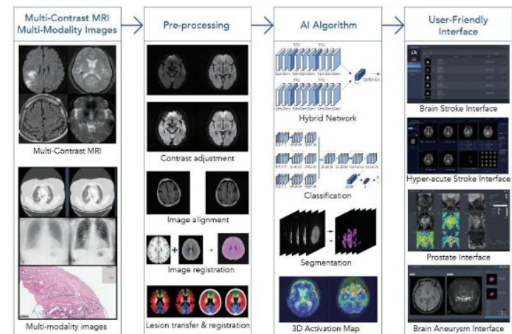
올인원 'AIHuB' 플랫폼 기반 인공지능 솔루션 구조
