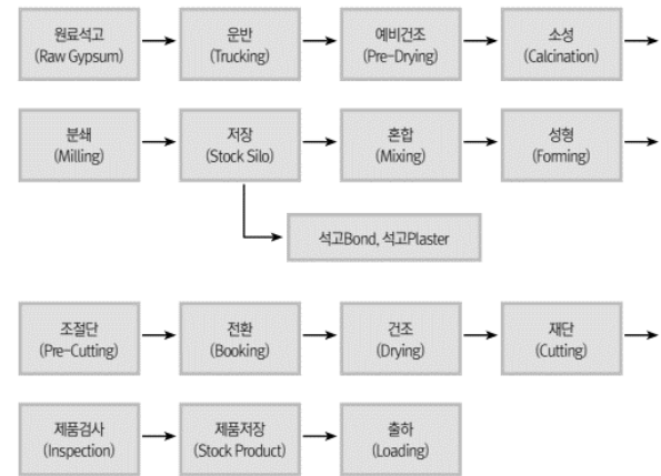
그림 2. 석고보드 제조공정도
