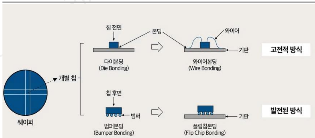
그림1 본딩 방식 비교(Die Bonding vs Flip chip Bonding)
