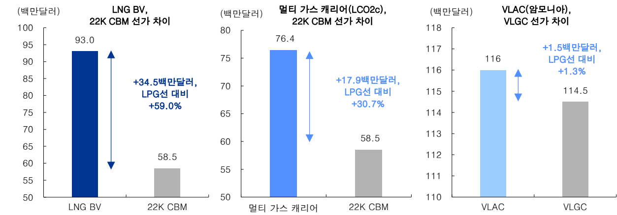
그림 2. 일반 LPG선과 멀티 가스 캐리어(LCO2c), LNG BV 가격 비교: 고수익성 탱크 비중 확대에 따른 믹스 개선 효과 전망
