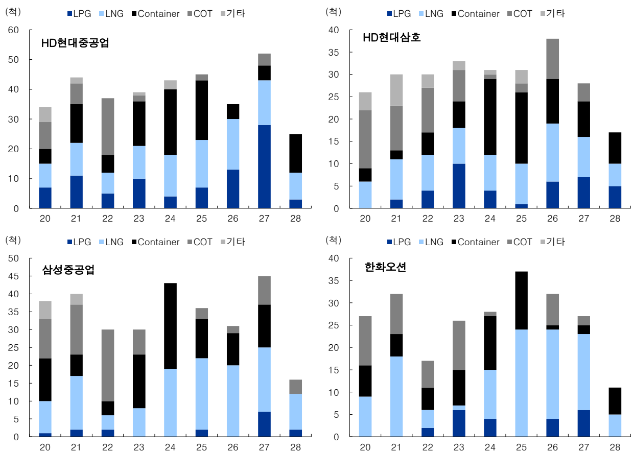
그림 17. 한국 대형 조선사 선종별 인도 일정: HD현대중공업 가스선 비중 가장 높음
