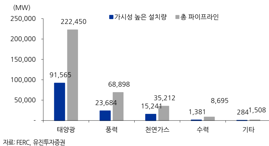
도표 3. 미국 2025~2027년 발전원별 신규 설치 예상
