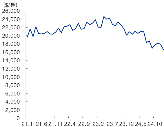
그림 3. 국내 탄소섬유 가격 추이
