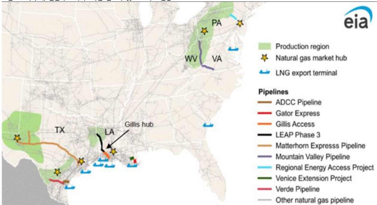
그림17. 미국 내 천연가스 파이프라인 인프라 및 프로젝트 현황
