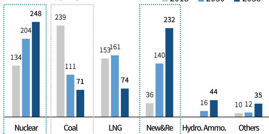
발전원별 발전량(TWh)
