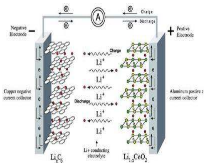
이차전지 구조
