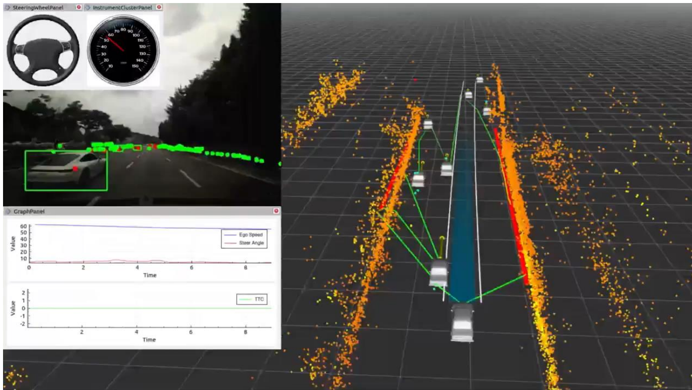
당사 Sensor Fusion (4D Imaging Radar + Camera) 시연
