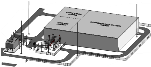
e-STATCOM
