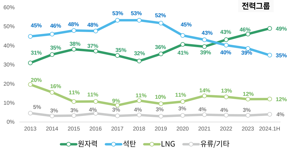
연도별 발전설비 (2013-2024.6) 1
