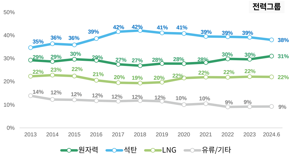
연도별 발전설비 (2013-2024.6) 1
