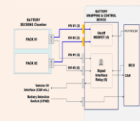
e-Mobility 시스템
