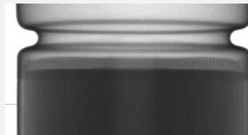
원통형 배터리
