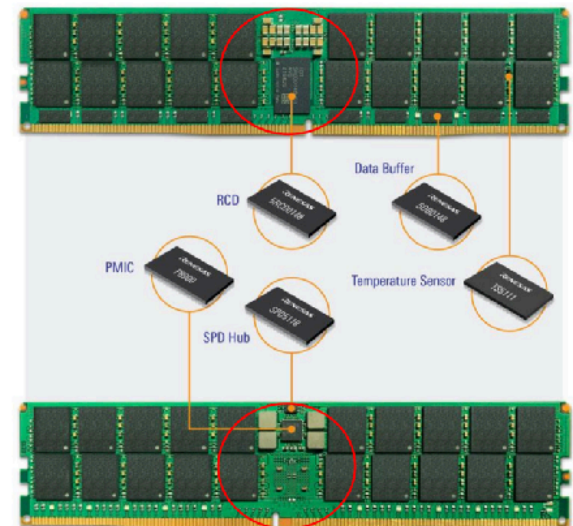
DDR5 구조도: 필요 반도체 증가
