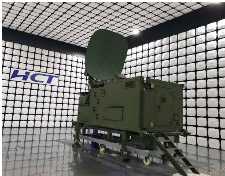
[ 에이치시티의 방산분야 EMC 인증시험 모습 ]
