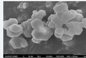
SEM of LOTAN-2MS1000
