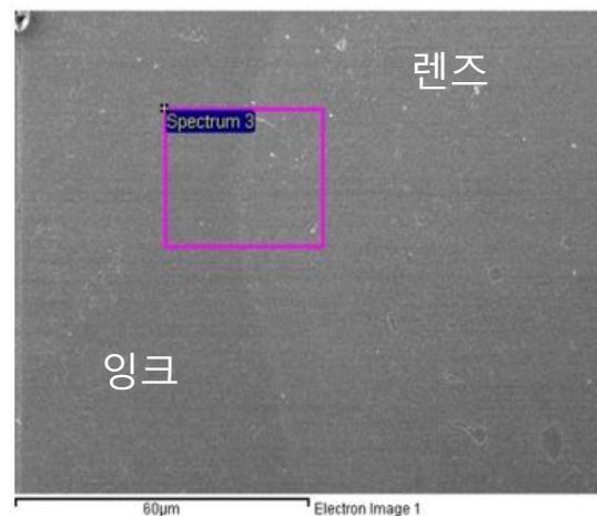
EDS
